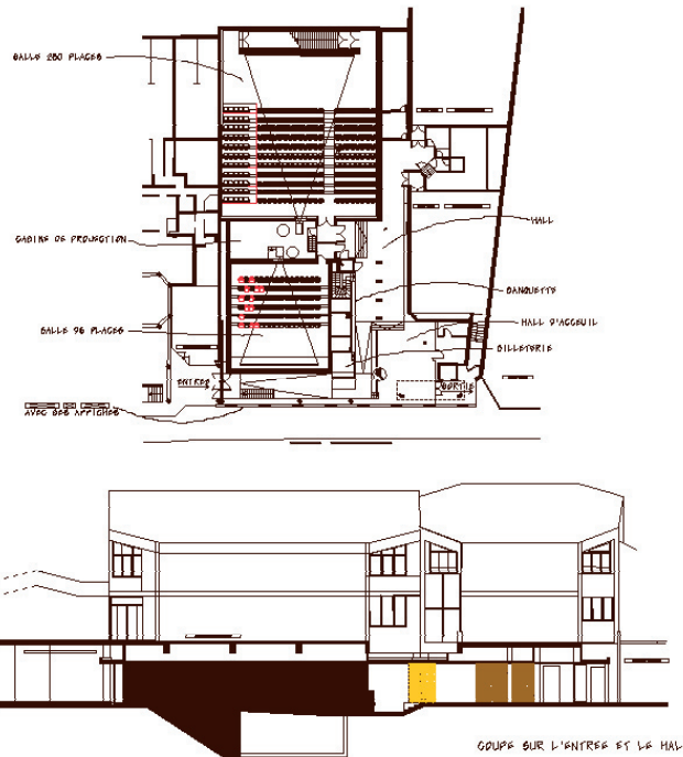
Coupes
